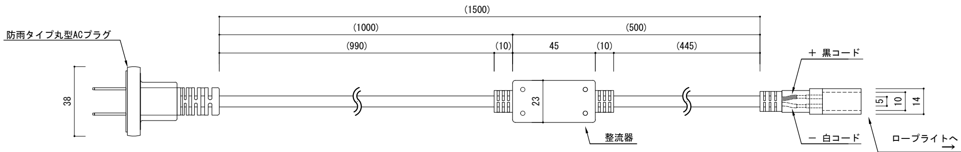
上面図
