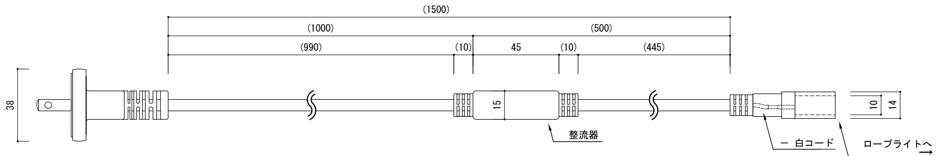
側面図
