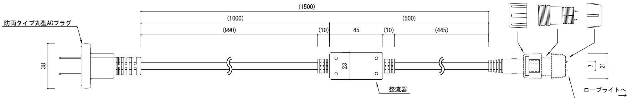
上面図
