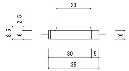
側面拡大図
