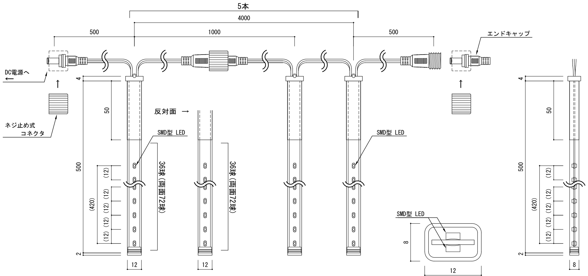
正面図
