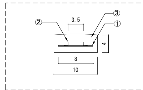
断面拡大図
