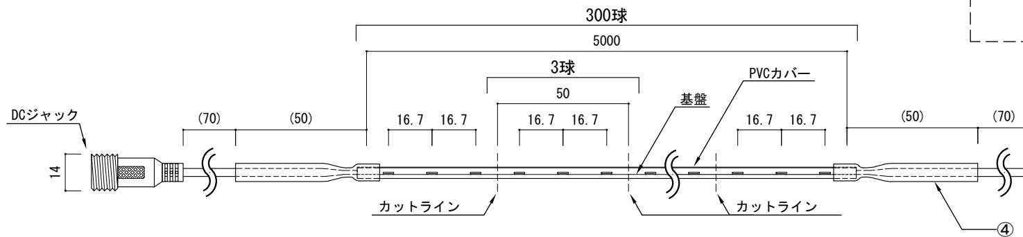
側面図
