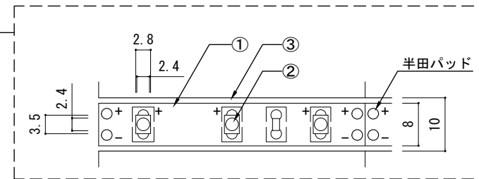
拡大図
