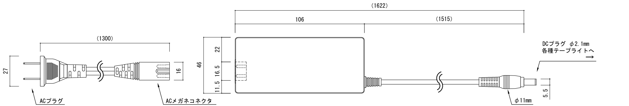
上面図
