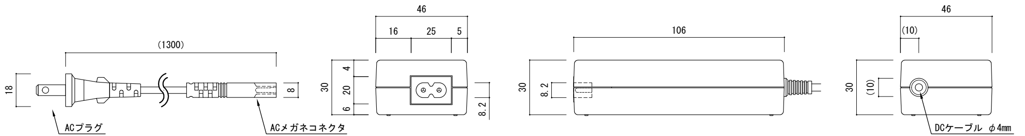
側面図
