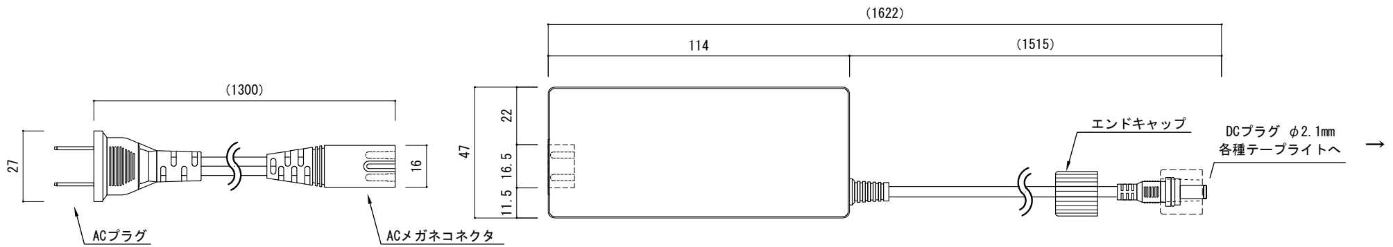
上面図
