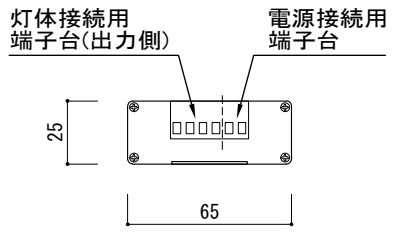
側面図 3
