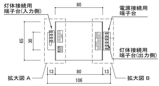
上面図
