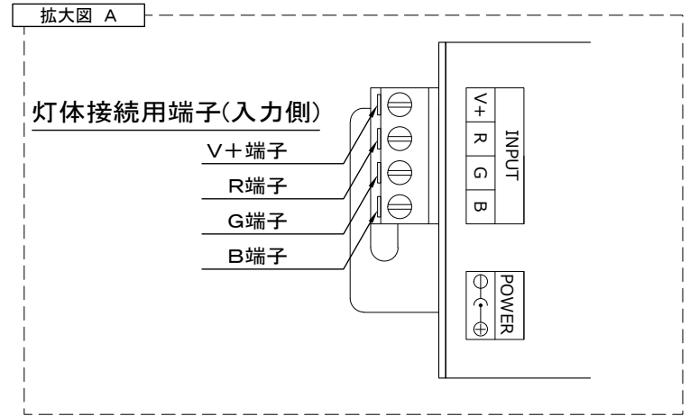
端子台 拡大図
