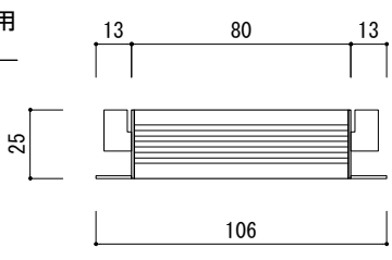
側面図 2
