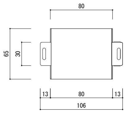
底面図
