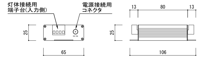
側面図 1
