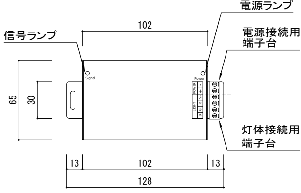
上面図
