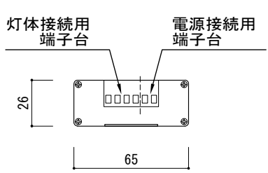
側面図 3
