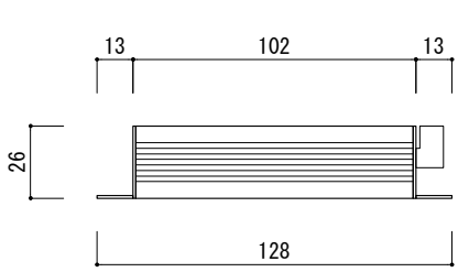
側面図 2
