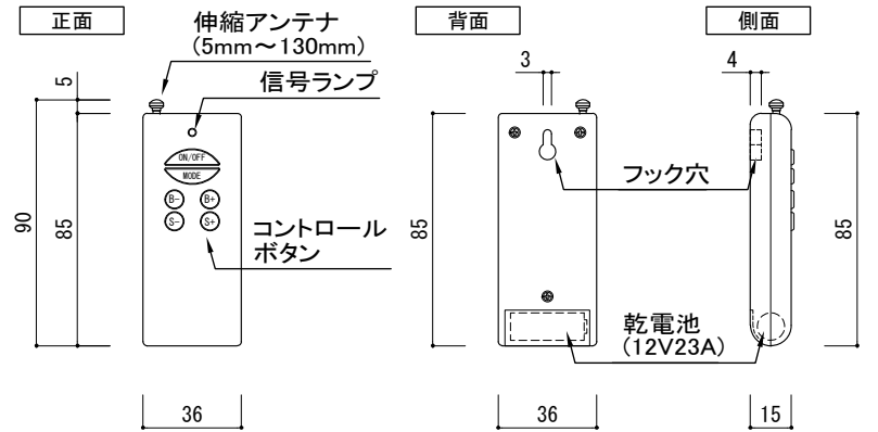
付属リモコン (非防水)
