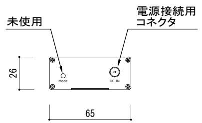
側面図 1
