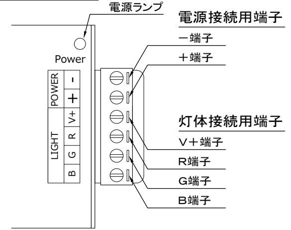
端子台 拡大図
