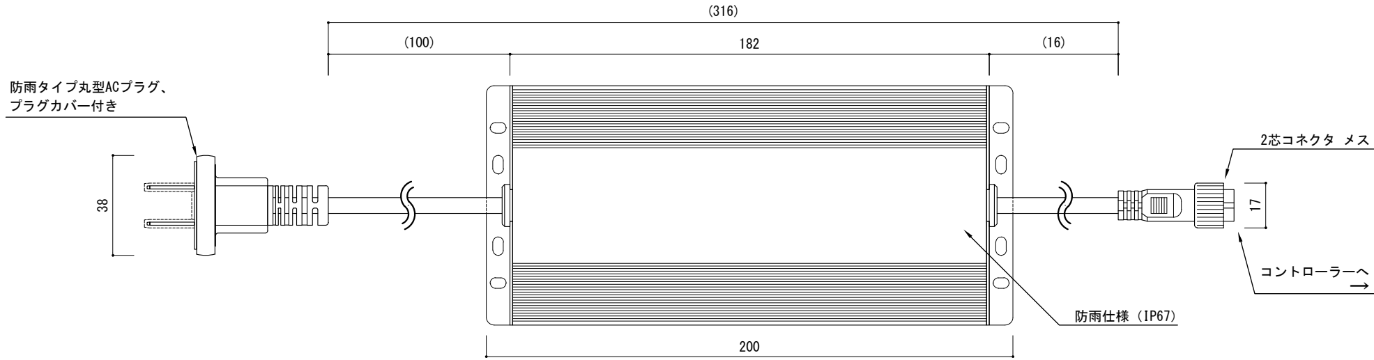
上面図
