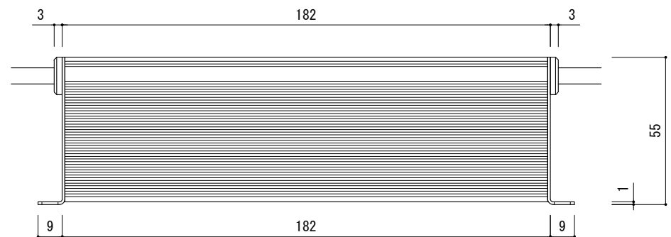
側面図
