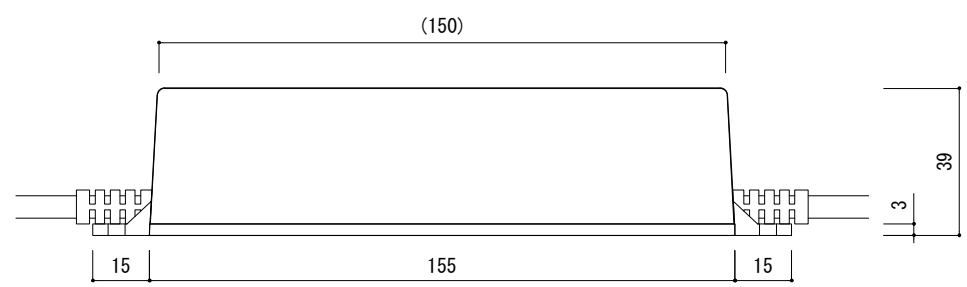
側面図
