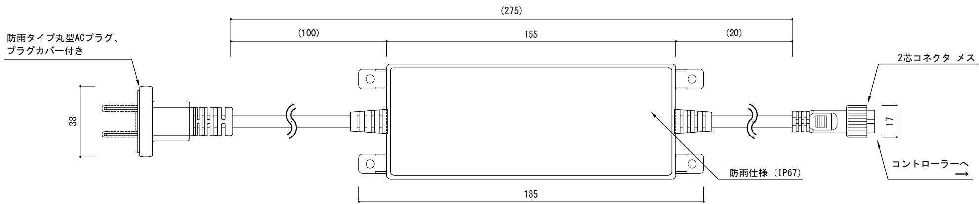
上面図
