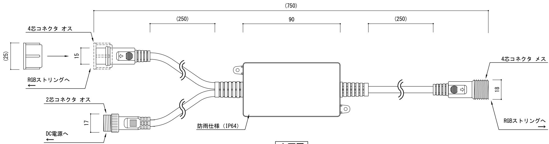
上面図
