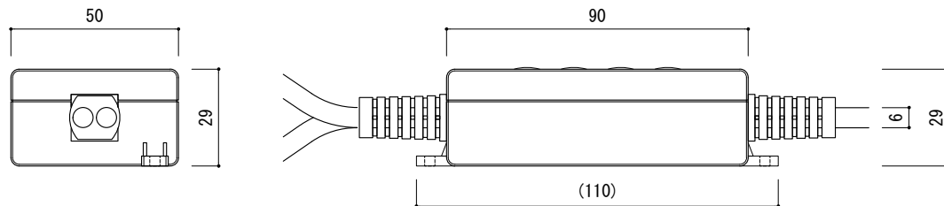
側面図
