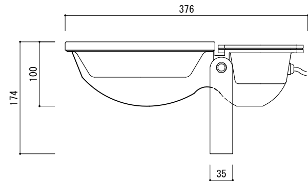
側面図 2
