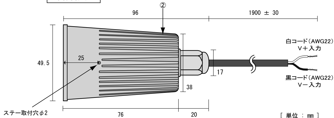
本体側面図
