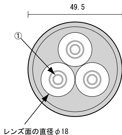
本体正面図
